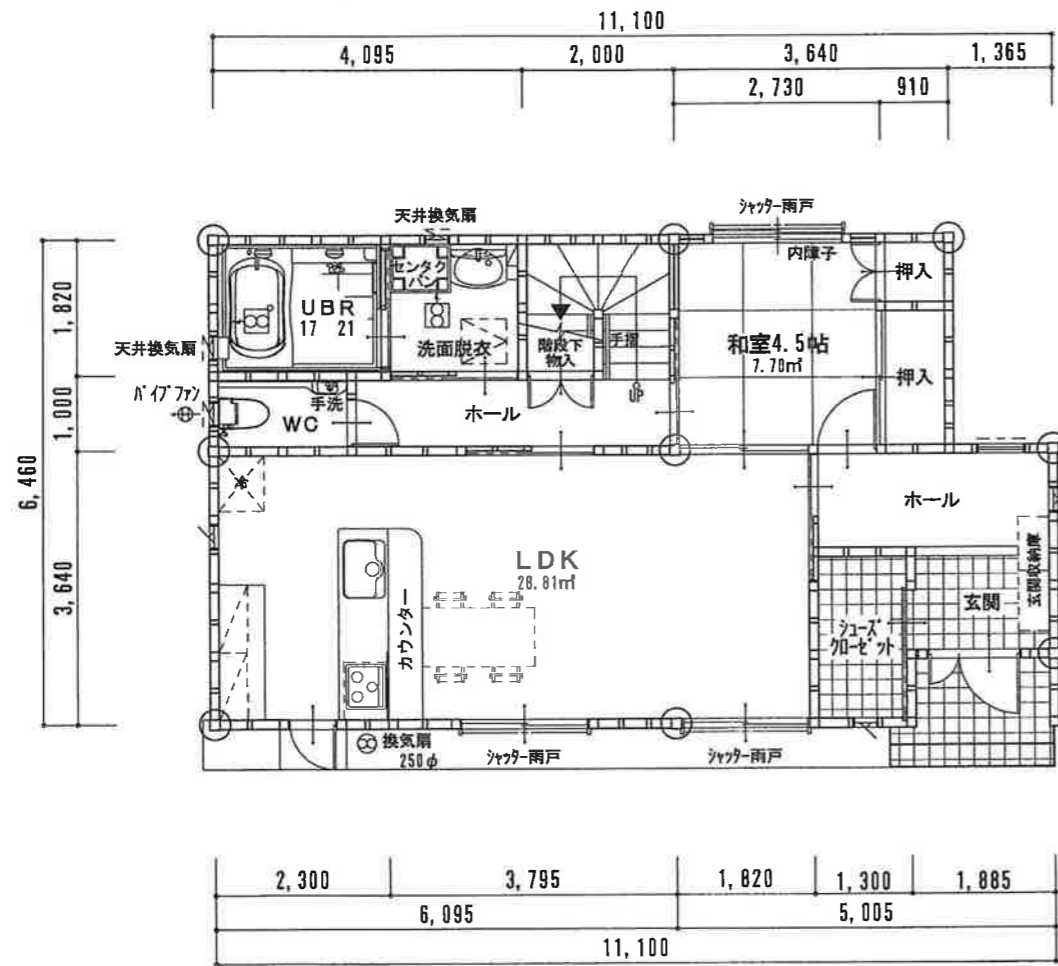
② 1階平面図 S=1/100
