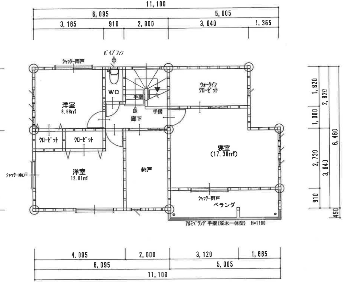
② 2階平面図 S=1/100
